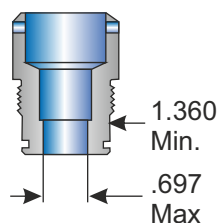
Orifice Sub
